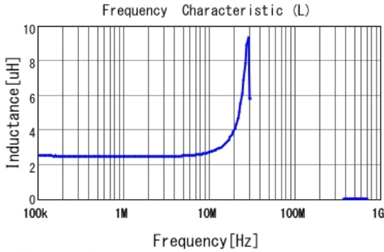
■ FDVE0640-H-2R2M L
