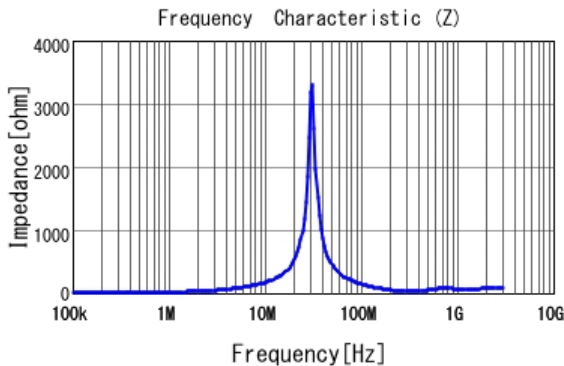
■ FDVE0640-H-2R2M |Z|
