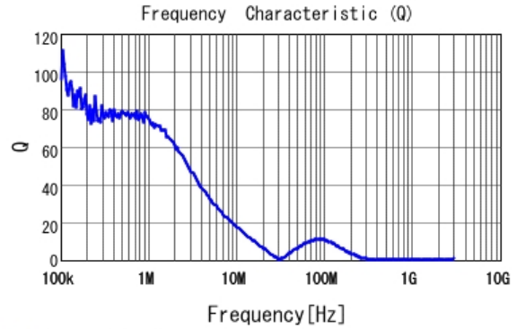
■ FDVE0640-H-2R2M Q
