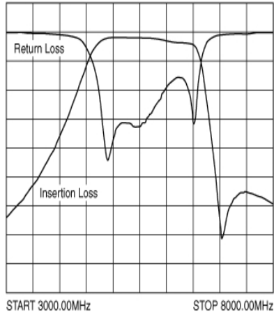
频率特性
