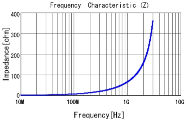
LQG15WH10NG02 |Z|
