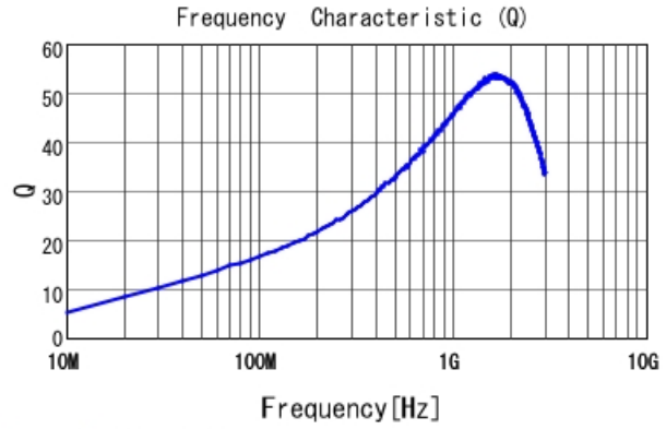
LQG15WH10NG02 Q
