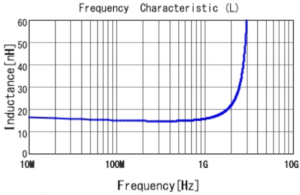
LQG15WH15NG02 L
