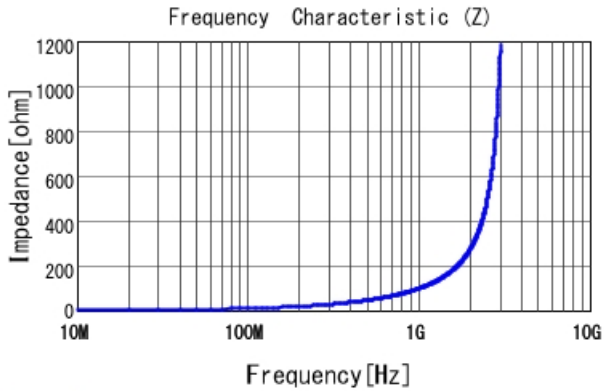
LQG15WH15NG02 |Z|
