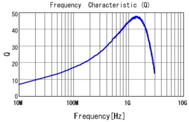
LQG15WH15NG02 Q
