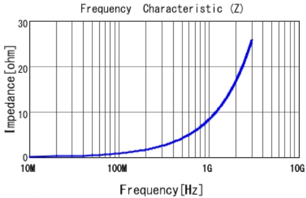
LQG15WH1N3B02 |Z|
