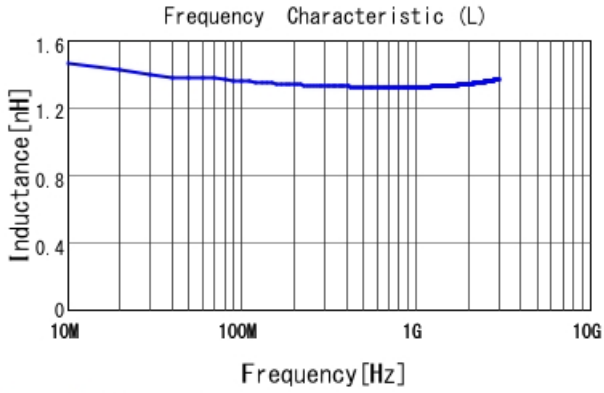
LQG15WH1N3B02 L
