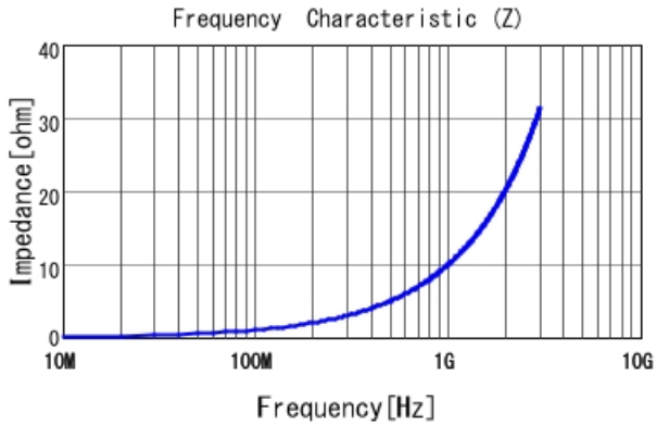
LQG15WH1N6B02 |Z|
