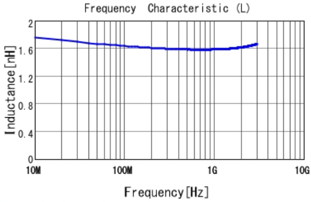
LQG15WH1N6B02 L
