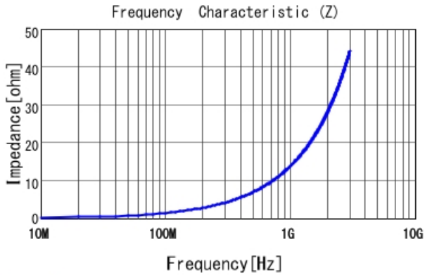
LQG15WH2N2B02 |Z|
