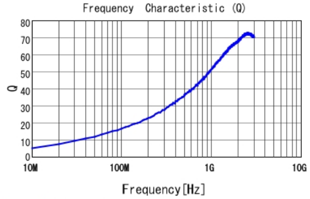
LQG15WH4N3B02 Q
