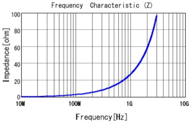
LQG15WH4N3B02 |Z|
