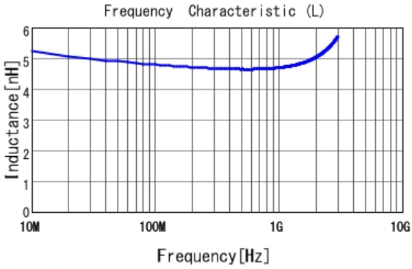
LQG15WH4N7B02 L
