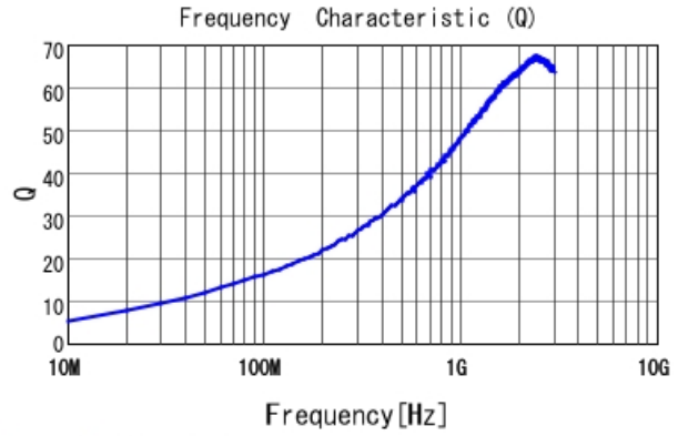
LQG15WH4N7B02 Q
