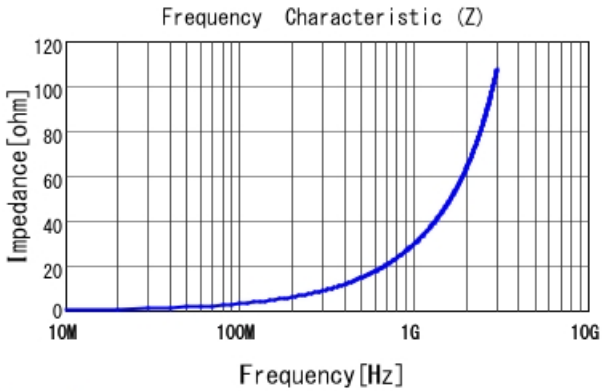
LQG15WH4N7B02 |Z|
