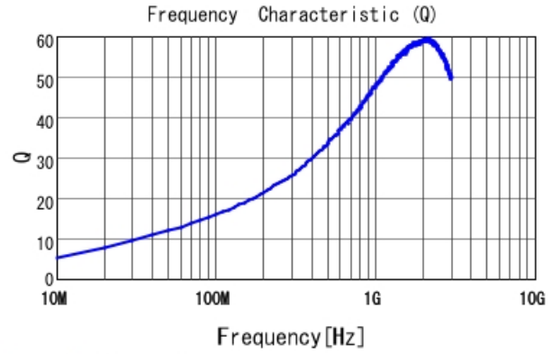
LQG15WH8N2G02 Q
