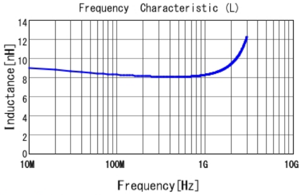
LQG15WH8N2G02 L
