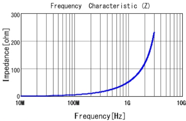
LQG15WH8N2G02 |Z|
