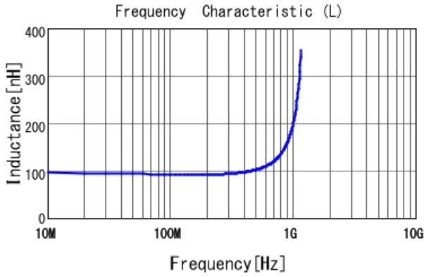
LQG15WH91NG02 L
