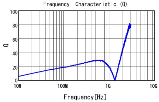
LQG15WH91NG02 Q
