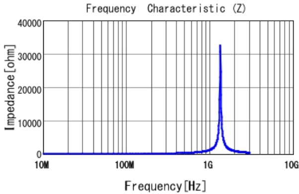
LQG15WH91NG02 |Z|
