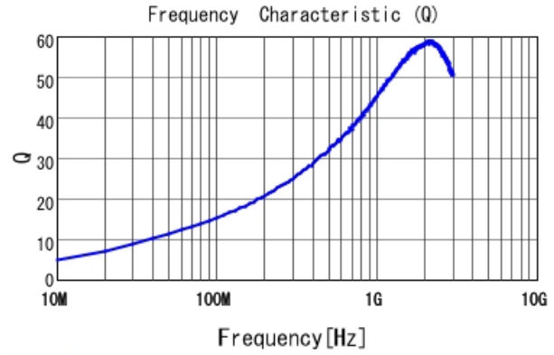
LQG15WZ6N2B02 Q
