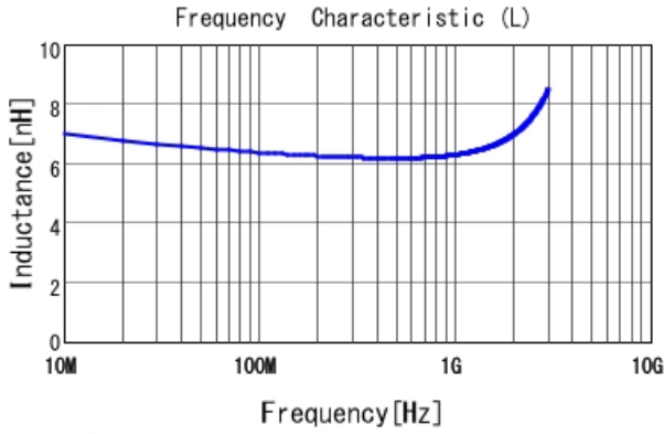
LQG15WZ6N2B02 L
