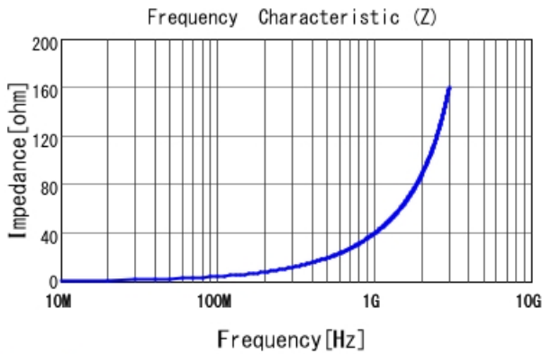
LQG15WZ6N2B02 |Z|
