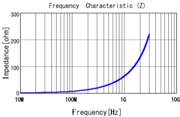
LQW04AN10NJ00 |Z|
