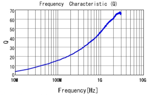
LQW04AN10NJ00 Q
