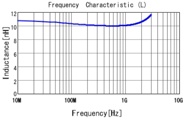
LQW04AN10NJ00 L
