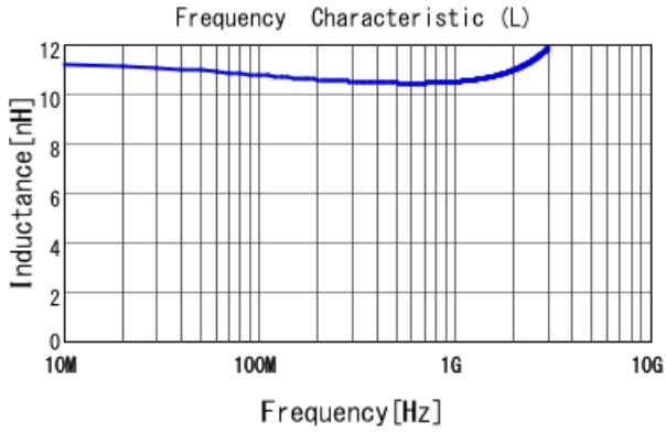
LQW04AN11NJ00 L
