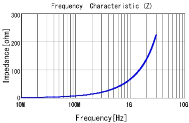
LQW04AN11NJ00 |Z|
