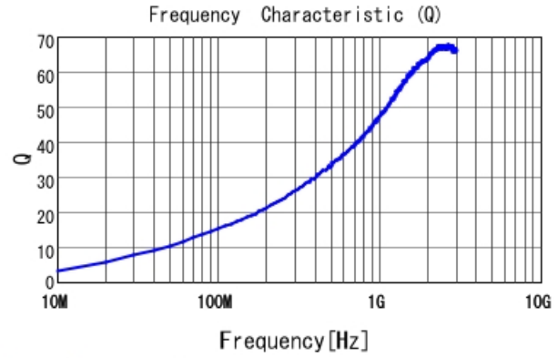
LQW04AN11NJ00 Q
