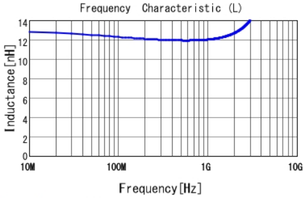
LQW04AN12NJ00 L
