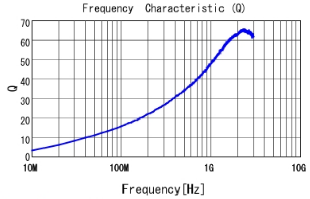
LQW04AN12NJ00 Q
