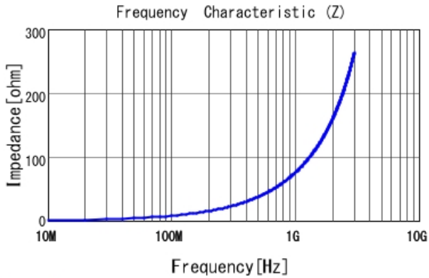
LQW04AN12NJ00 |Z|
