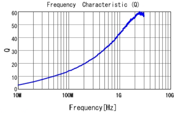
LQW04AN14NH00 Q
