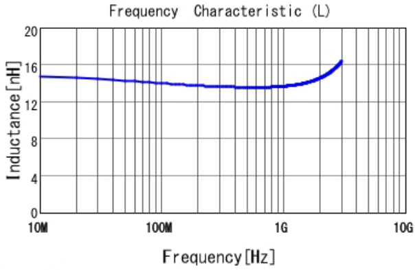
LQW04AN14NH00 L
