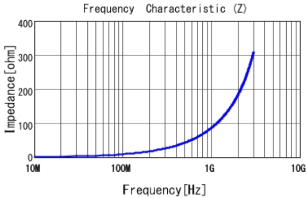
LQW04AN14NH00 |Z|
