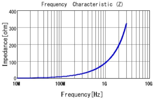
LQW04AN15NJ00 |Z|
