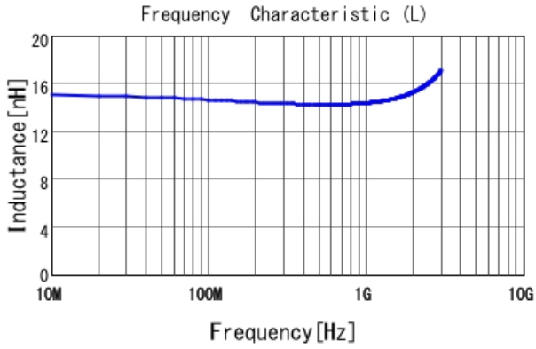
LQW04AN15NJ00 L
