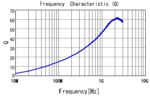
LQW04AN15NJ00 Q
