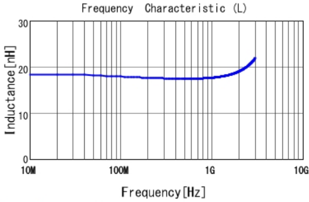
LQW04AN18NJ00 L
