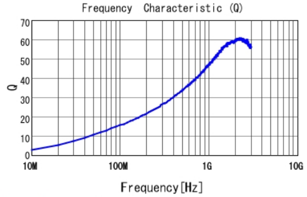
LQW04AN18NJ00 Q
