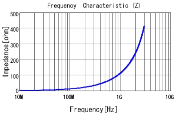
LQW04AN18NJ00 |Z|
