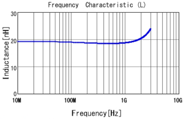
LQW04AN19NH00 L
