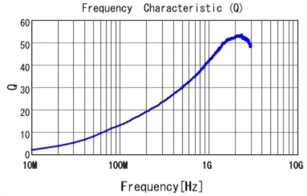
LQW04AN19NH00 Q
