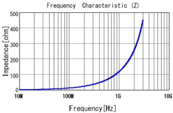
LQW04AN19NH00 |Z|
