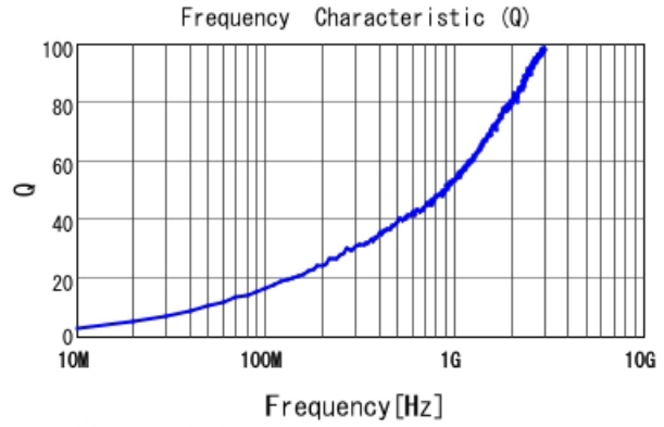
LQW04AN1N1C00 Q
