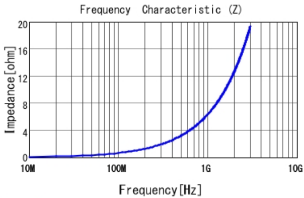
LQW04AN1N1C00 |Z|
