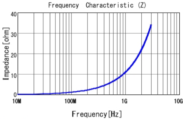
LQW04AN1N6C00 |Z|
