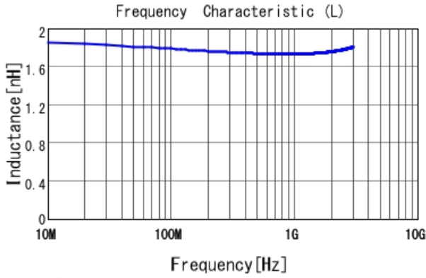
LQW04AN1N6C00 L
