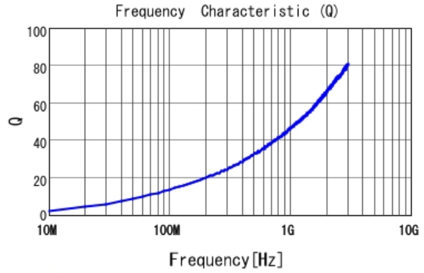
LQW04AN1N6C00 Q
