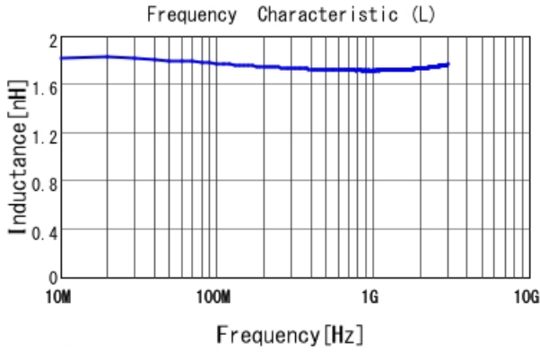
LQW04AN1N8C00 L
