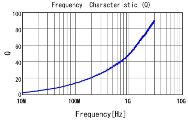
LQW04AN1N8C00 Q
