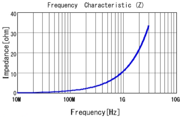
LQW04AN1N8C00 |Z|
