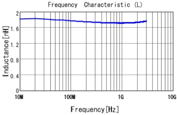
LQW04AN1N8D00 L
