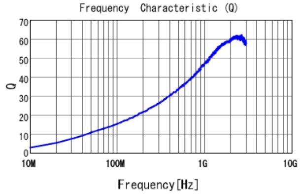
LQW04AN20NH00 Q
