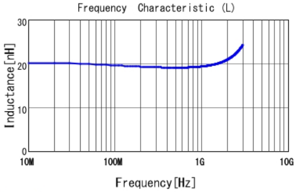
LQW04AN20NH00 L
