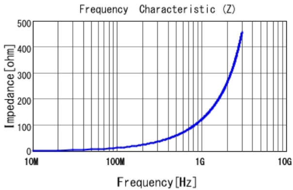
LQW04AN20NH00 |Z|
