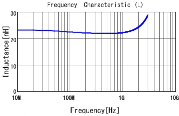
LQW04AN22NH00 L
