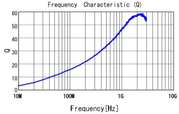
LQW04AN22NH00 Q
