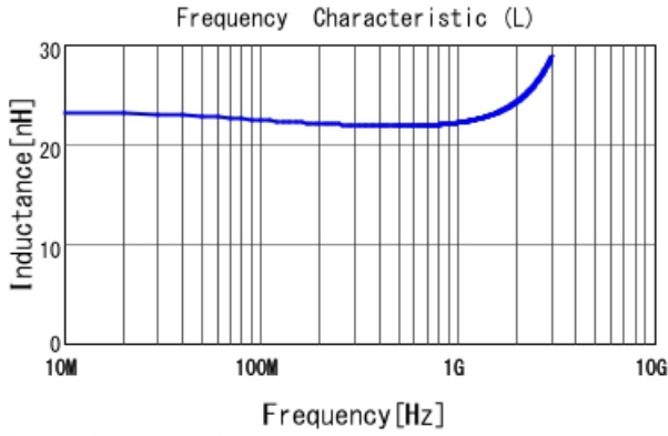
LQW04AN22NJ00 L
