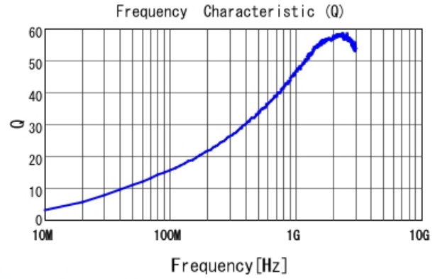
LQW04AN22NJ00 Q
