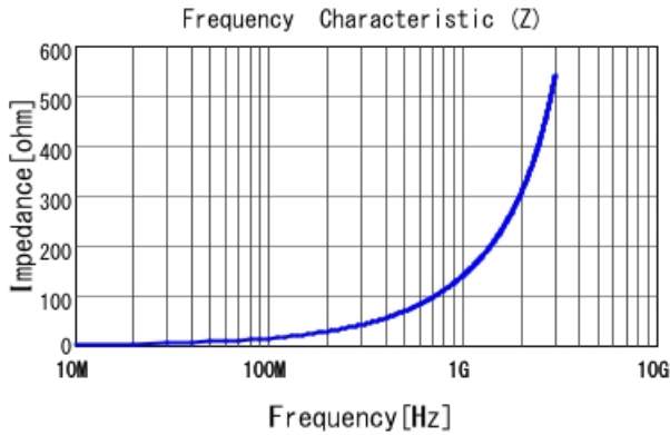
LQW04AN22NJ00 |Z|
