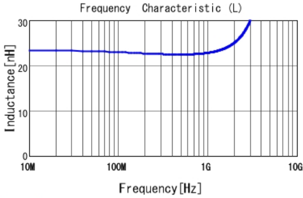
LQW04AN23NH00 L
