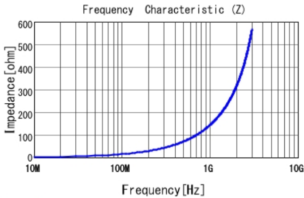
LQW04AN23NH00 |Z|
