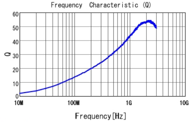
LQW04AN23NH00 Q
