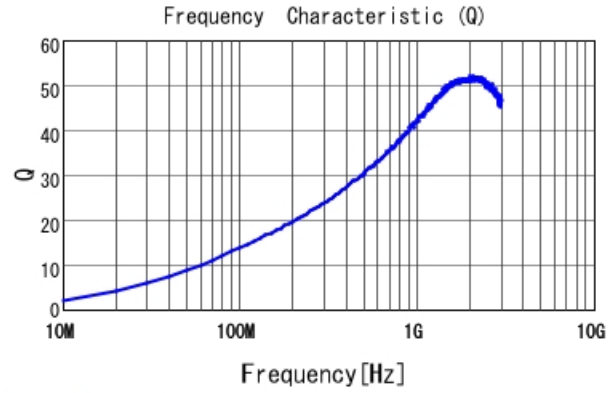
LQW04AN24NH00 Q
