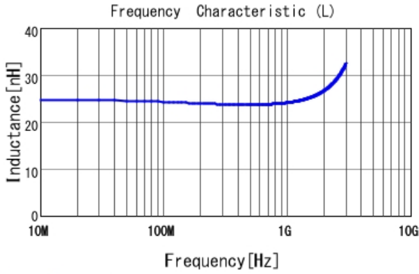
LQW04AN24NH00 L
