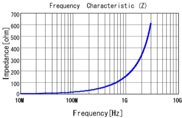
LQW04AN24NH00 |Z|
