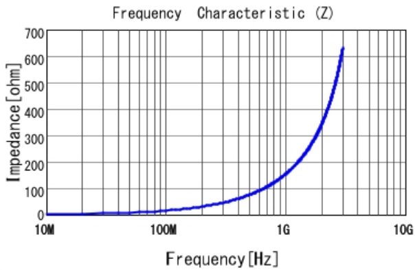
LQW04AN25NH00 |Z|
