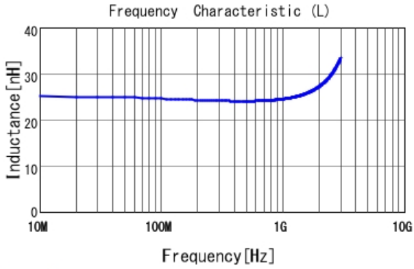
LQW04AN25NH00 L
