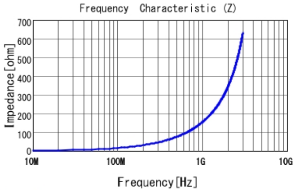
LQW04AN25NJ00 |Z|
