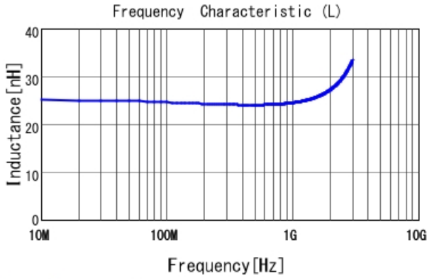
LQW04AN25NJ00 L
