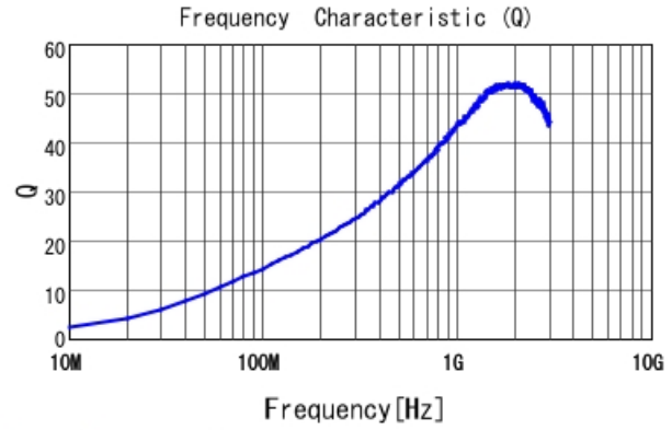
LQW04AN25NJ00 Q
