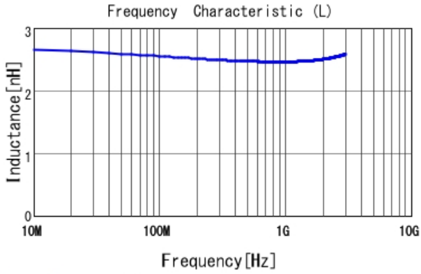
LQW04AN2N4C00 L
