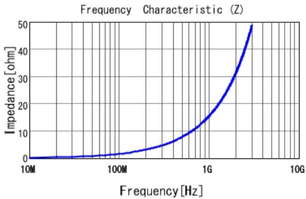
LQW04AN2N4C00 |Z|
