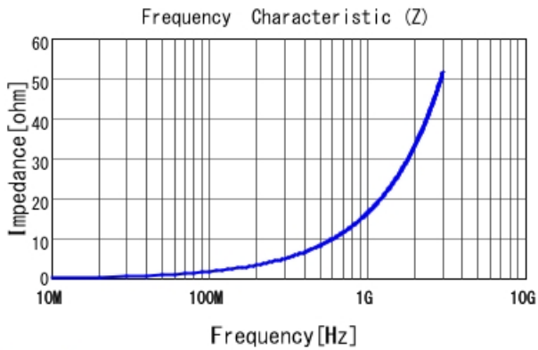
LQW04AN2N6C00 |Z|
