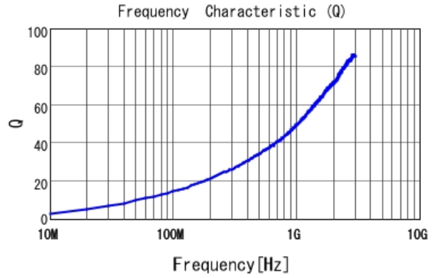
LQW04AN2N6C00 Q
