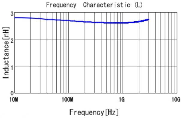
LQW04AN2N6C00 L
