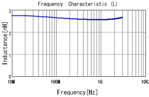
LQW04AN2N7C00 L
