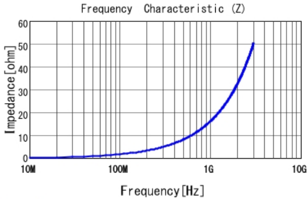
LQW04AN2N7C00 |Z|
