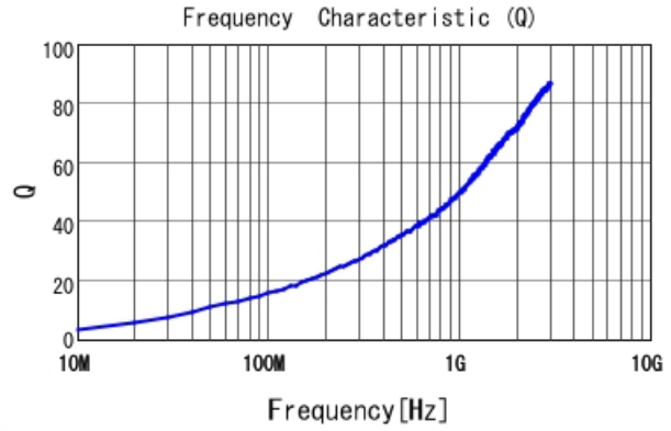
LQW04AN2N7D00 Q
