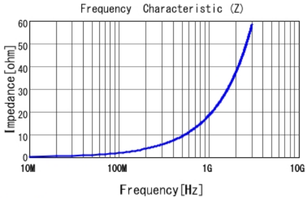
LQW04AN2N9C00 |Z|
