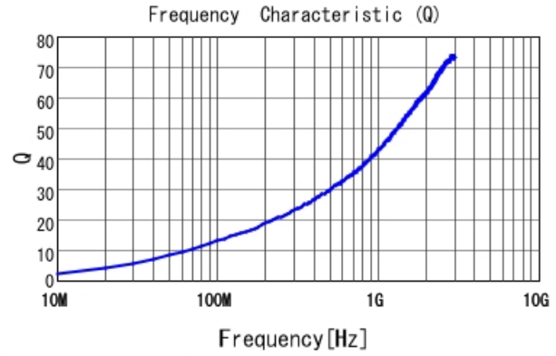
LQW04AN2N9C00 Q
