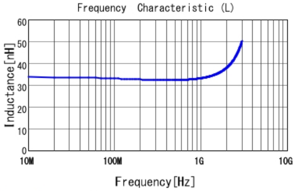
LQW04AN33NJ00 L
