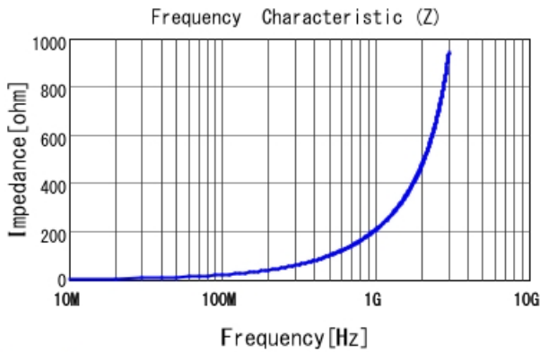
LQW04AN33NJ00 |Z|
