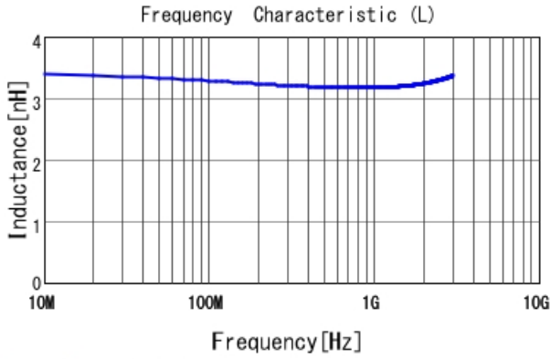
LQW04AN3N1C00 L
