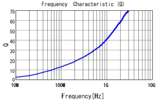
LQW04AN3N1C00 Q
