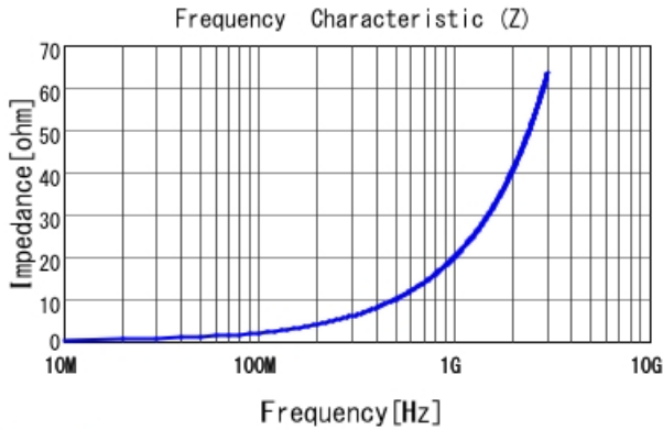
LQW04AN3N1C00 |Z|
