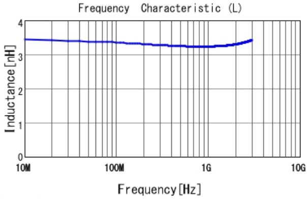
LQW04AN3N2C00 L
