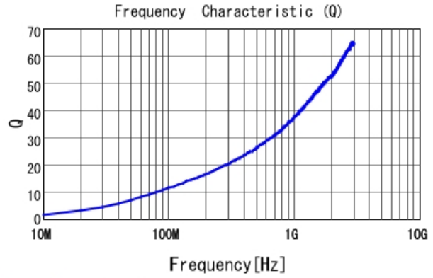
LQW04AN3N2C00 Q
