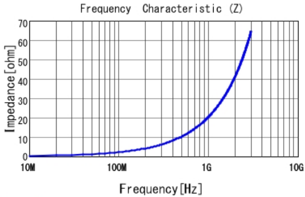
LQW04AN3N2C00 |Z|
