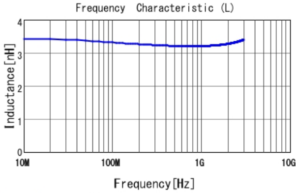
LQW04AN3N3C00 L
