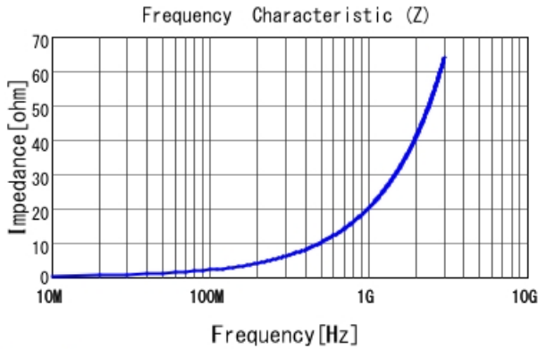
LQW04AN3N3C00 |Z|
