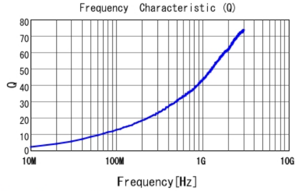
LQW04AN3N3C00 Q
