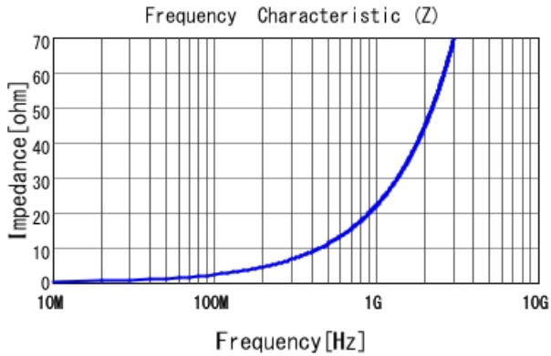
LQW04AN3N6C00 |Z|
