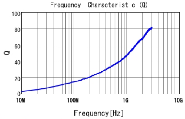
LQW04AN3N6C00 Q
