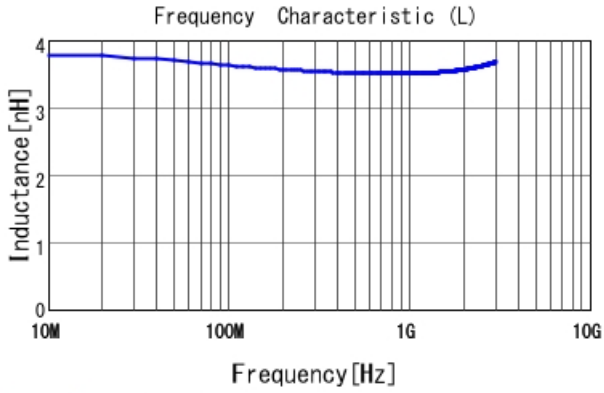
LQW04AN3N6C00 L
