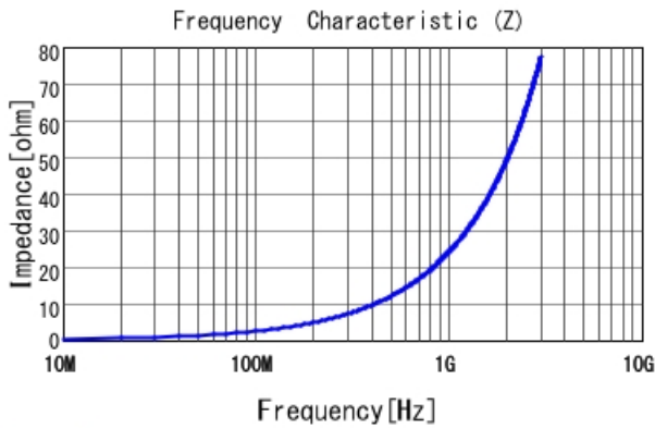
LQW04AN3N8C00 |Z|
