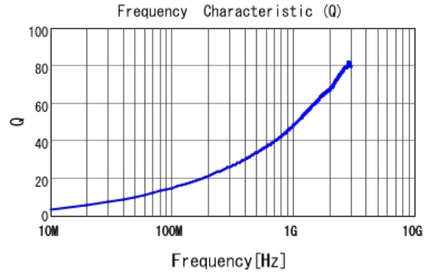
LQW04AN3N8C00 Q
