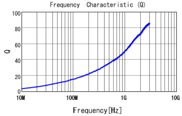
LQW04AN3N9D00 Q
