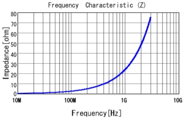
LQW04AN3N9D00 |Z|
