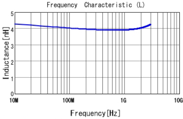
LQW04AN4N0D00 L
