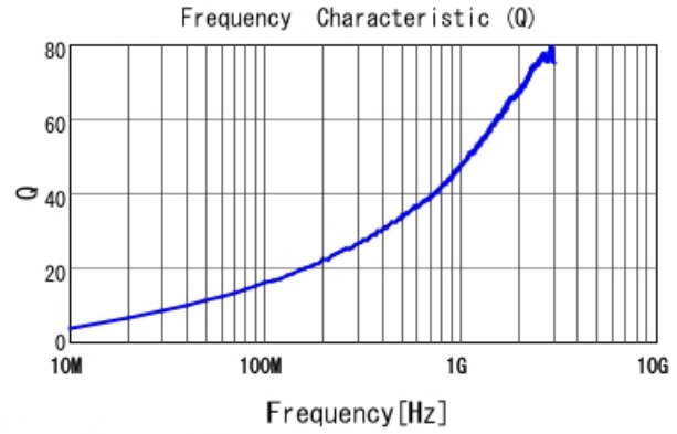
LQW04AN4N0D00 Q
