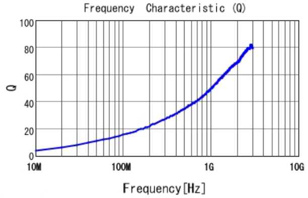
LQW04AN4N1C00 Q
