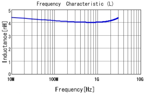
LQW04AN4N1C00 L
