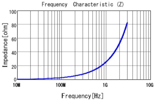
LQW04AN4N1C00 |Z|
