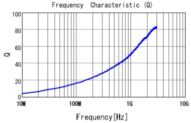
LQW04AN4N3C00 Q
