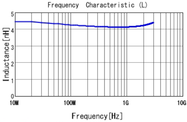
LQW04AN4N3C00 L
