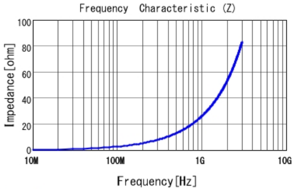
LQW04AN4N3C00 |Z|
