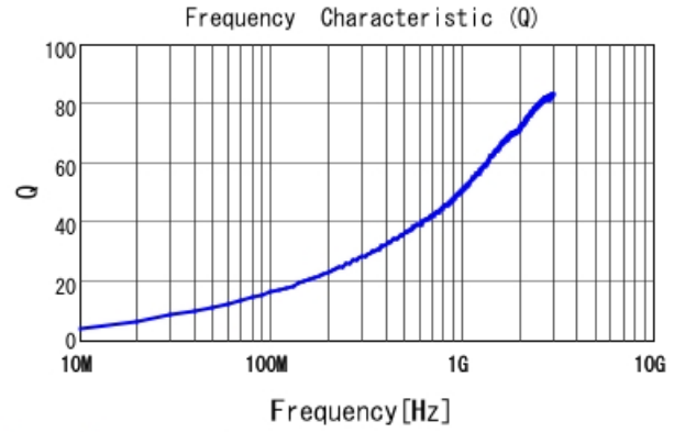
LQW04AN4N3D00 Q
