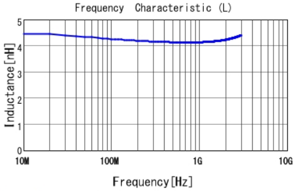
LQW04AN4N3D00 L
