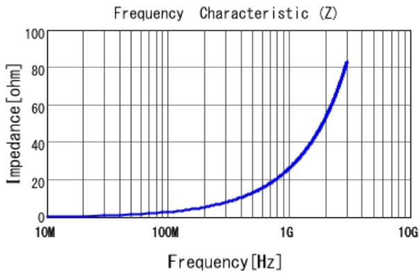
LQW04AN4N3D00 |Z|
