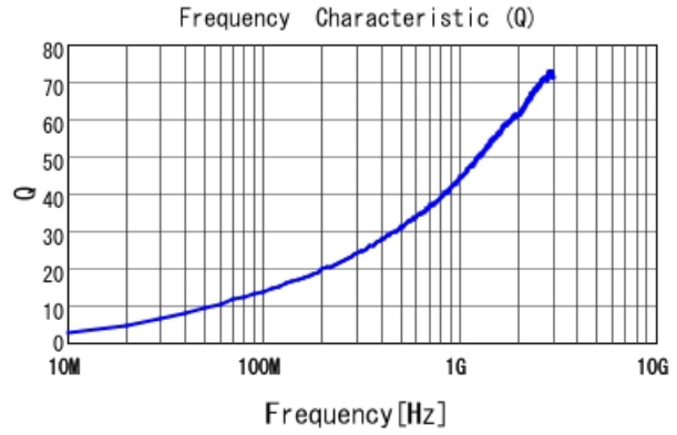
LQW04AN4N4C00 Q
