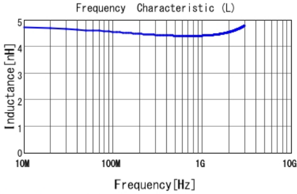
LQW04AN4N4C00 L
