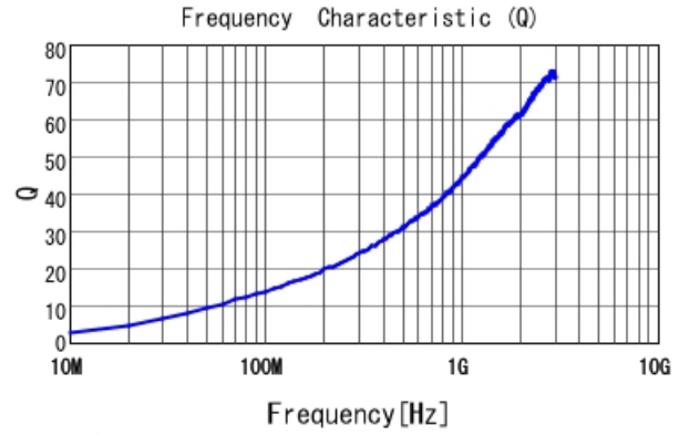
LQW04AN4N4D00 Q
