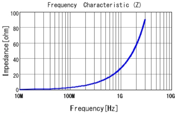
LQW04AN4N4D00 |Z|
