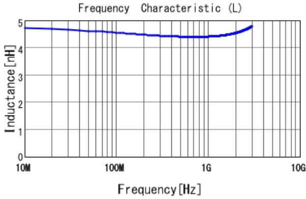
LQW04AN4N4D00 L
