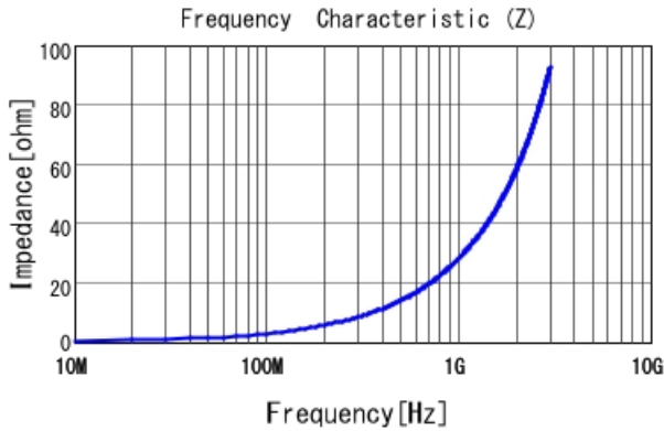
LQW04AN4N5C00 |Z|
