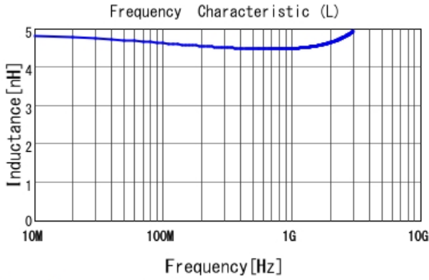
LQW04AN4N5C00 L
