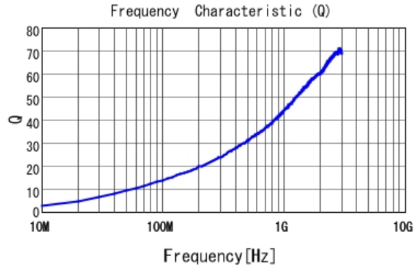
LQW04AN4N5C00 Q
