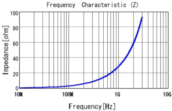
LQW04AN4N5D00 |Z|
