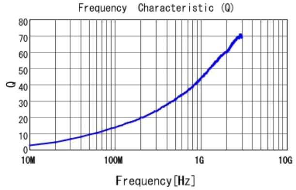
LQW04AN4N5D00 Q
