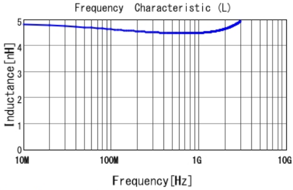
LQW04AN4N5D00 L
